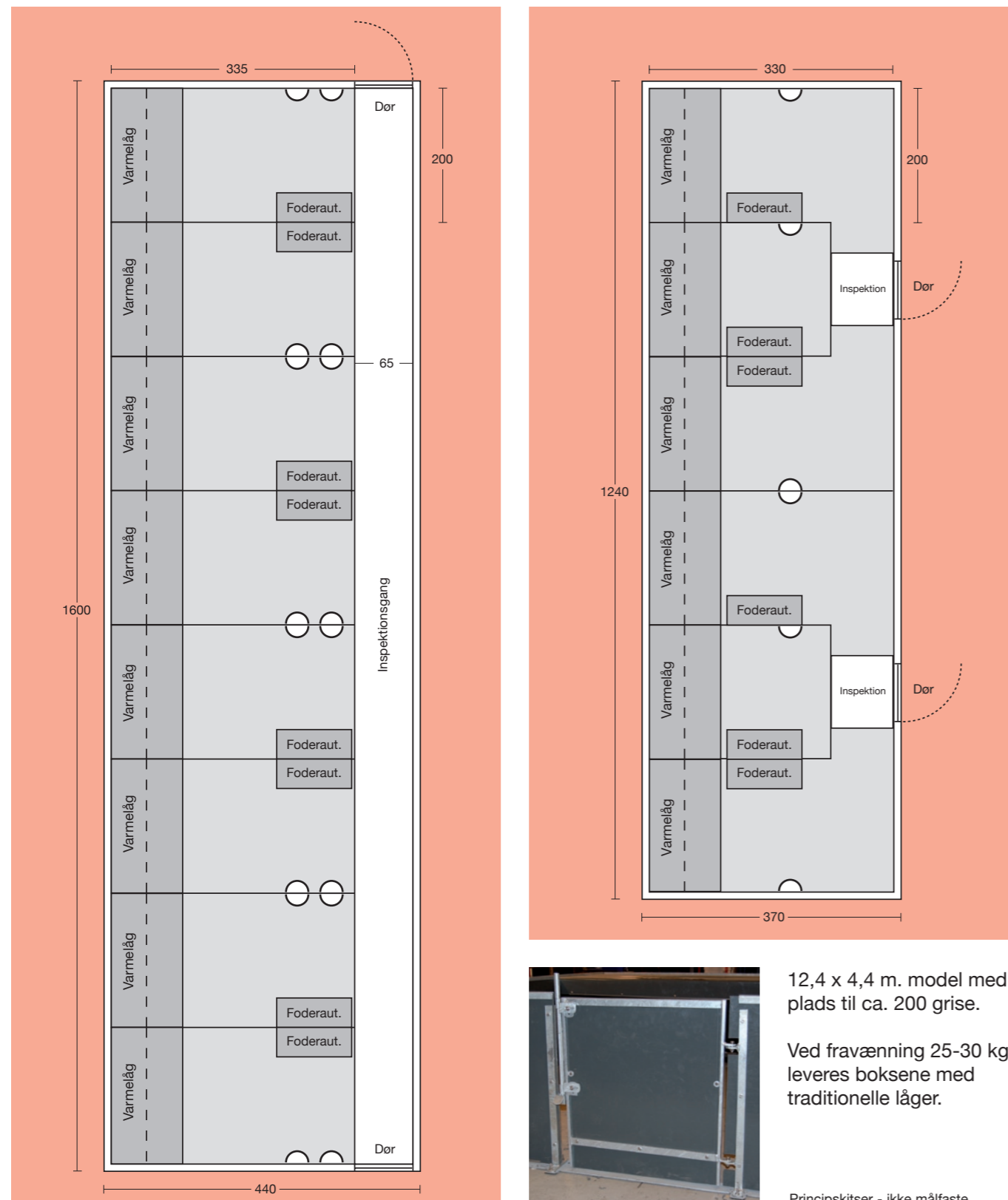
16,0 x 4,4 m. model med plads til ca. 250 grise.
